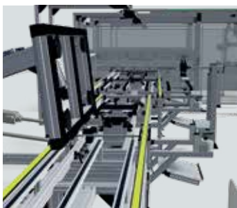
Montažna linija za fotovoltaične module z napravo za spajanje okvirjev
